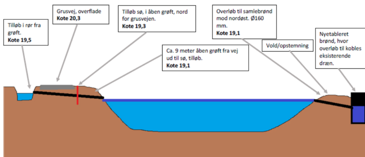
Bilag 6: Skitse, til- og fraløbskoter efter etablering
