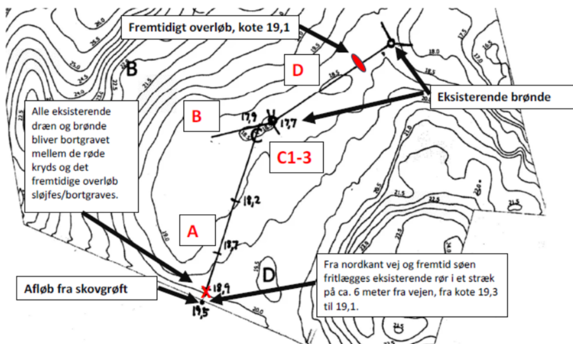
Bilag 4: Skitse, drænløb
